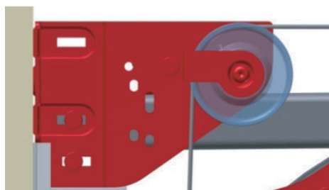
Kábeltartócsa 1. pozíció Cable pulley position 1
